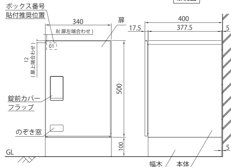
扉開図
