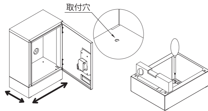
■取付穴ピッチ図
